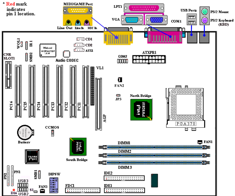
圖 1-1. SE6 主機板重要元件位置圖
