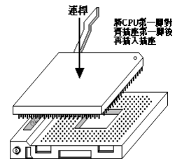
圖 2-4. 將處理器安裝到 Socket 370 插座
