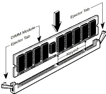
圖 2-6. 記憶體模組之安裝
