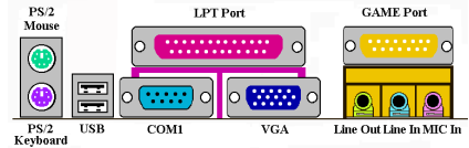
圖 2-11. 背板之連接器
