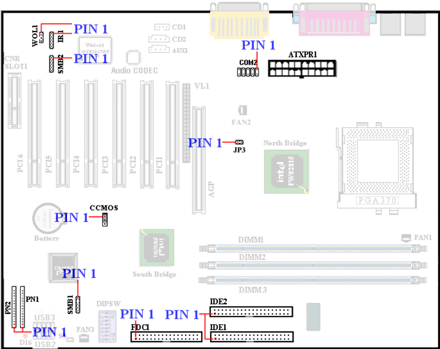
圖 2-7. SE6 所有的連接埠及接頭
