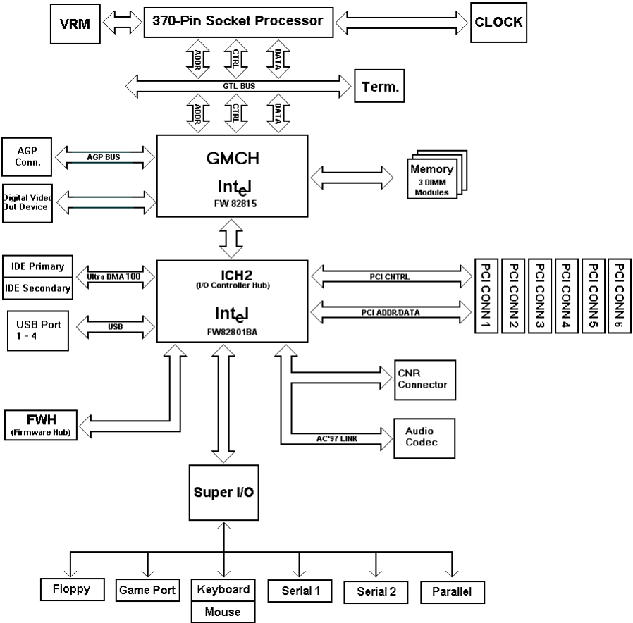
圖 1-2. INTEL 815E 晶片組之系統架構
