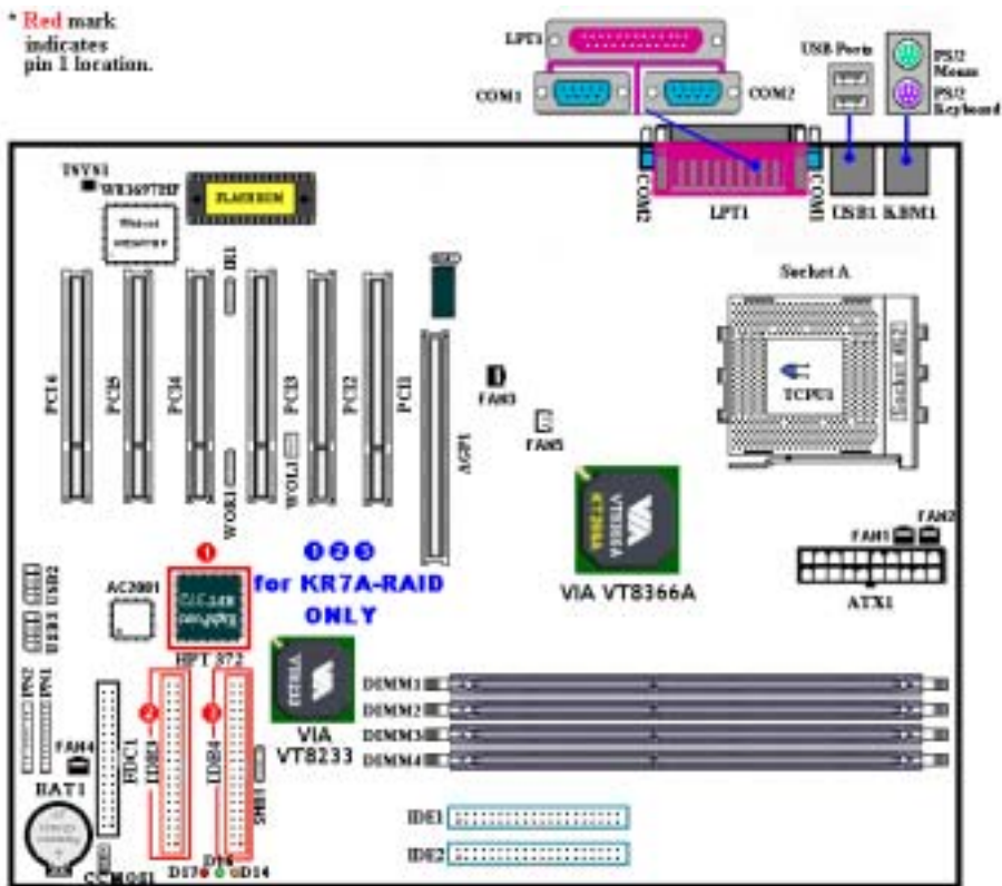
圖 1-1. KR7A/KR7A-RAID 主機板重要元件位置圖
