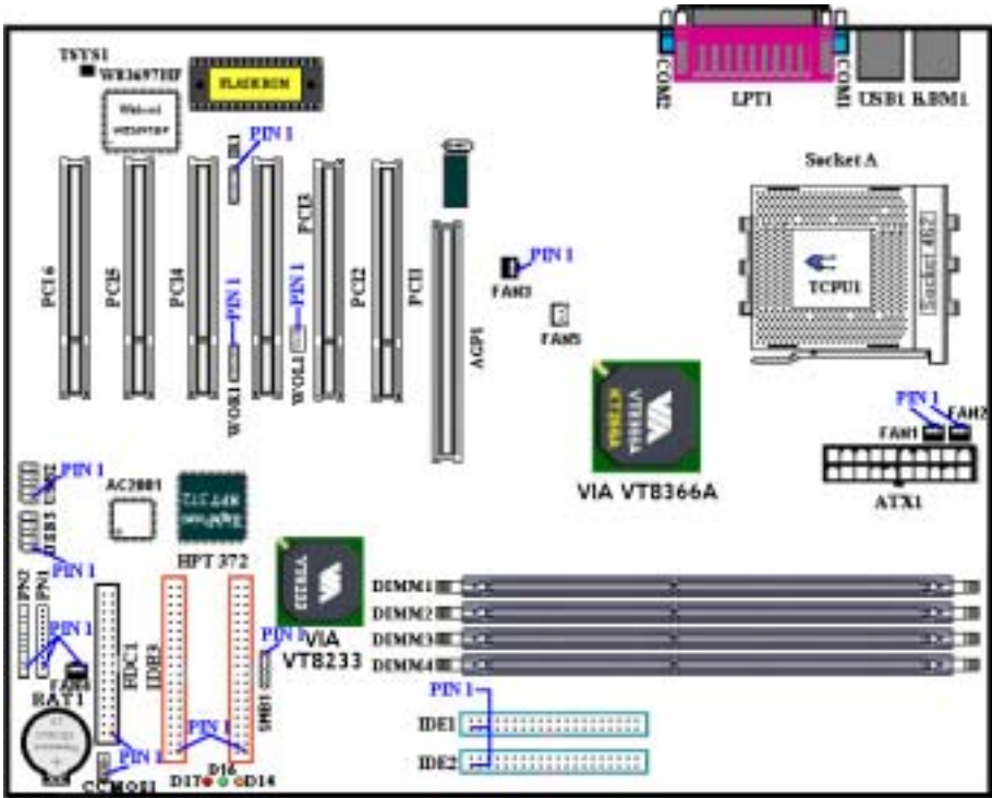
圖 2-7. KR7A/KR7A-RAID 主機板的所有連接埠和接頭
