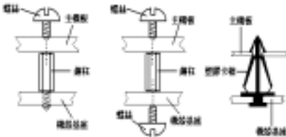
圖 2-2. 固定主機板至機殼的幾種方法
