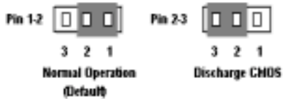
圖 2-8. CCMOS1 插帽的設定
