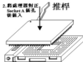
圖2-4. 將處理器安裝至Socket A之中
